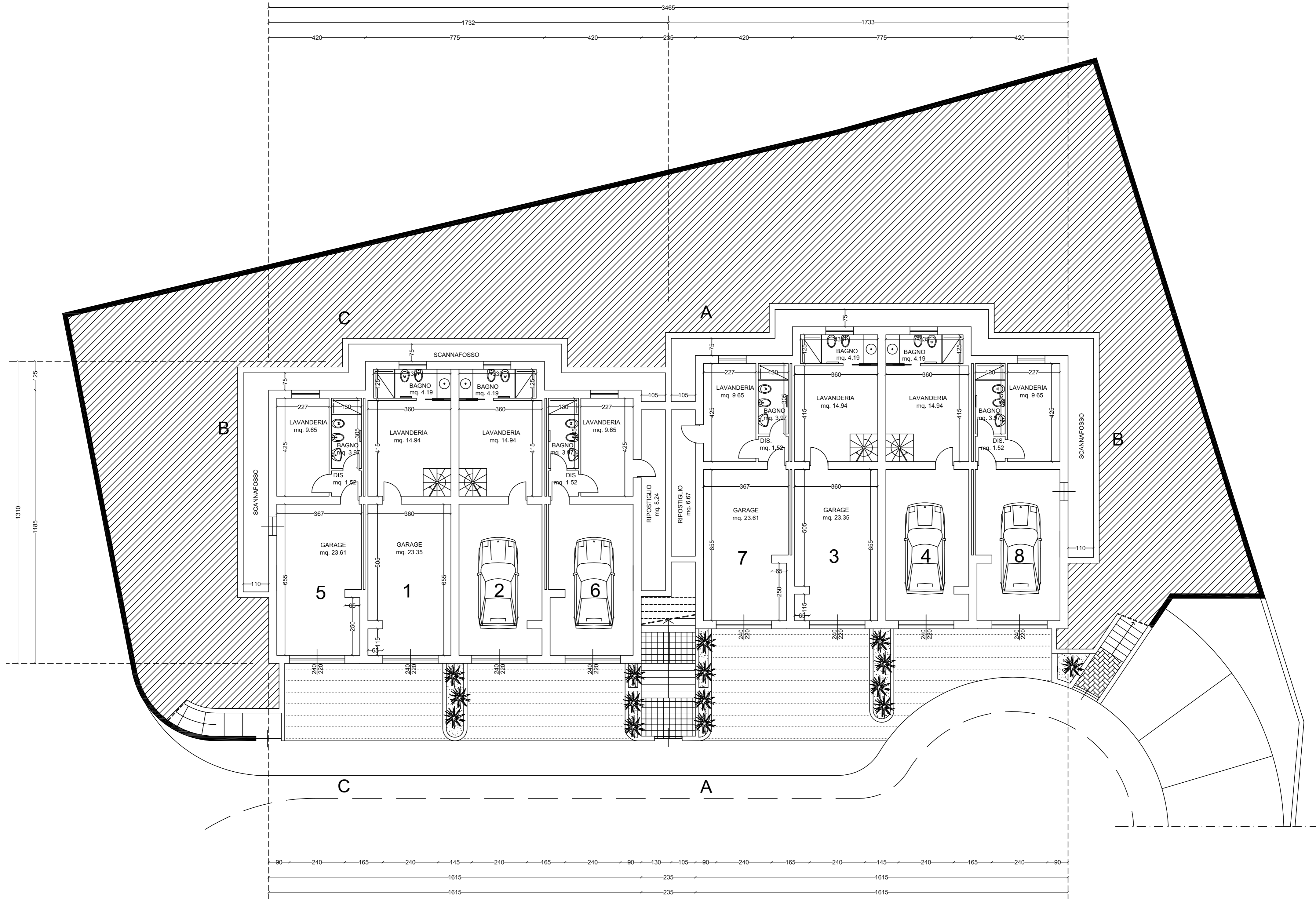
PIANTA PIANO SEMINTERRATO
