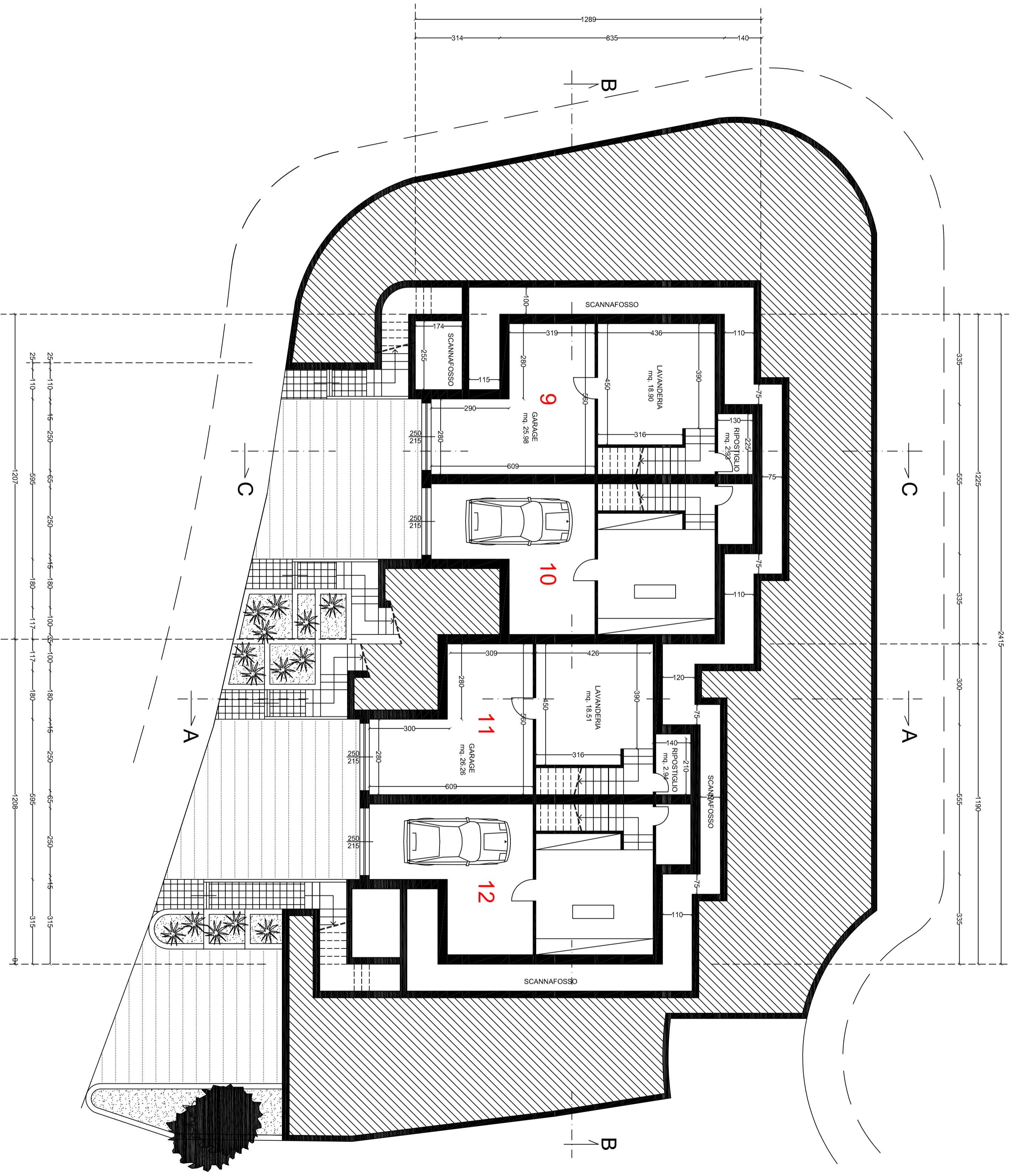
PIANTA PIANO SEMINTERRATO
